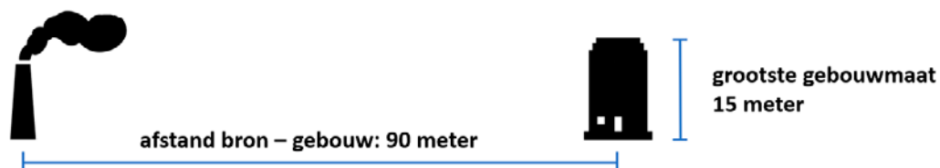
Figuur 4.4 De afstand tussen bron (losstaande schoorsteen) en gebouw is hier 6 maal de grootste gebouwmaat; gebouwinvloed moet hier in principe meegenomen worden.
