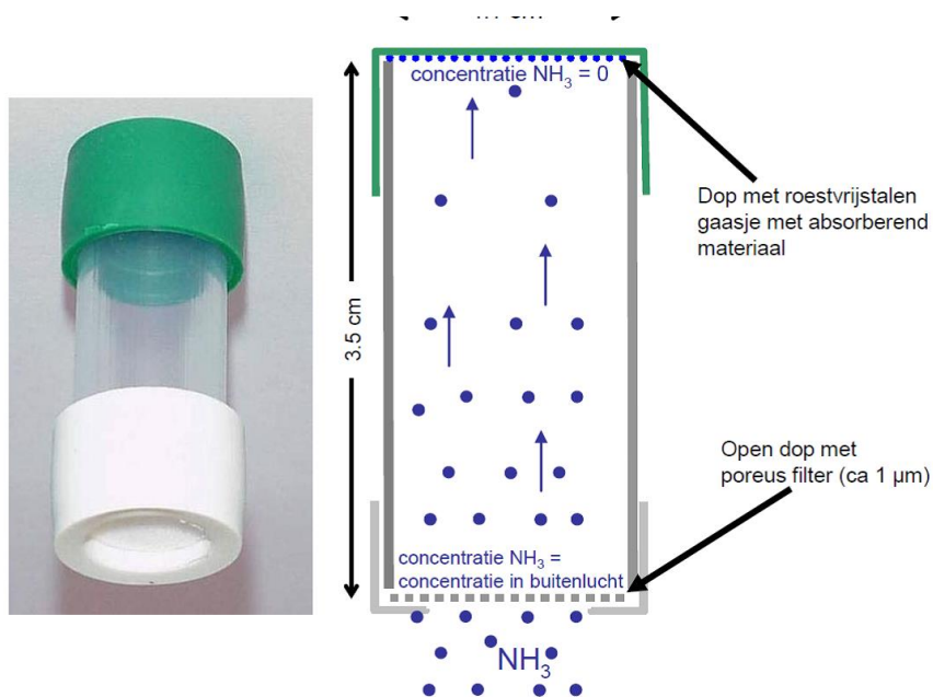
Figuur 4. Een Gradco-metbuisje, ook wel passieve sampler genoemd. Deze metingen worden samen met het LML gebruikt om maandgemiddelde ammoniakconcentraties te verkrijgen. Bron: https://www.rivm.nl/stikstof/mee-netten
