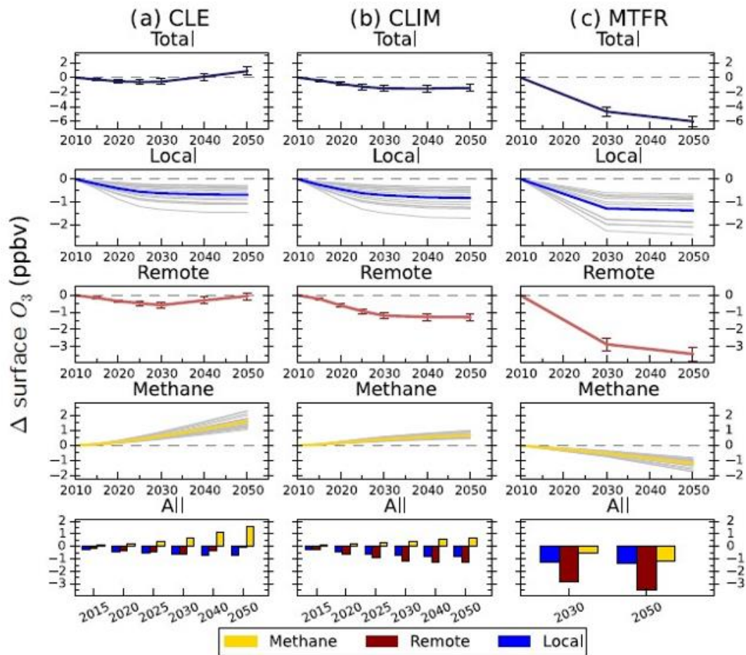
Bijlage Figuur 4: Totale jaarlijkse gemiddelde verandering in regionale O_3 concentraties aan het oppervlak in Europa (links) en de bijdrage van lokale (blauwe), afgelegen (rode) en methaan (geel) bronnen tussen 2010 en 2050 onder de CLE (a), CLIM (b) en MTFR (c) scenario's. Grijze lijnen op de lokale en methaanpanelen vertegenwoordigen individuele modelschattingen van O_3 -veranderingen, en tonen de spreiding in modelresponsen; ononderbroken lijnen tonen het gemiddelde van meerdere modellen. Foutbalken vertegenwoordigen 1 standaarddeviatie over het modelbereik. De laatste rij panelen toont de O_3 -respons van individuele bronnen die voor elk jaar samen zijn uitgezet. Uit Turnock, 2018.
