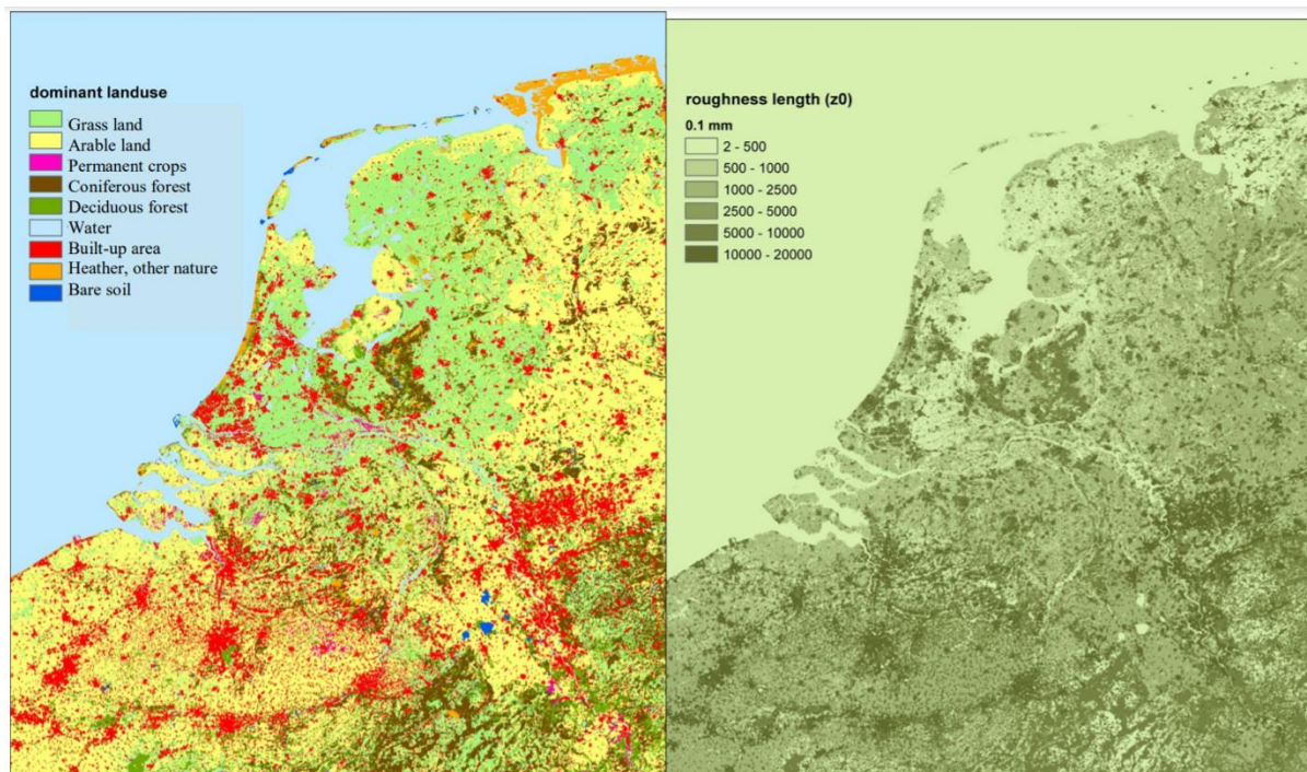
Figuur 39: Dominant landgebruik (volgens DEPAC) en ruwheidslengte op 250 bij 250 m 2 , afgeleid van LGN7 voor Nederland n CLC2006 voor België en Duitsland (volgens handleiding OPS).
